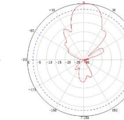
B2030019-V00 14dBi
