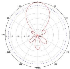
B2030017-V00 10dBi
