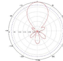
B2030018-V00 12dBi
