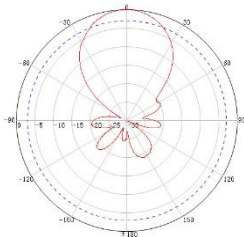
B2030016-V00 8dBi
